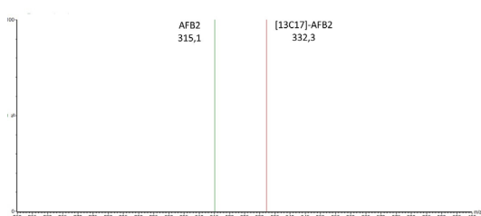
Spectre MS de l'Aflatoxine B2 et étalon LIB'UP® U-[ ^{13}\text{C}17 ]-Aflatoxine B2
