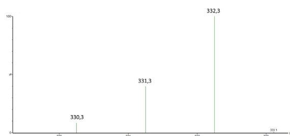
Spectre MS de l'étalon LIB'UP® U-[ ^{13}\text{C}17 ]-Aflatoxine B2
