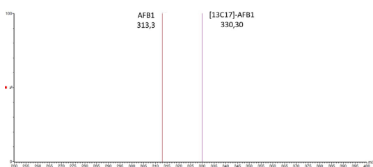
Spectre MS de l'Aflatoxine B1 et étalon LIB'UP® U-[ ^{13}\text{C}17 ]-Aflatoxine B1
