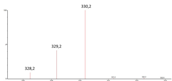
Spectre MS de l'étalon LIB'UP® U-[ ^{13}\text{C}17 ]-Aflatoxine B1
